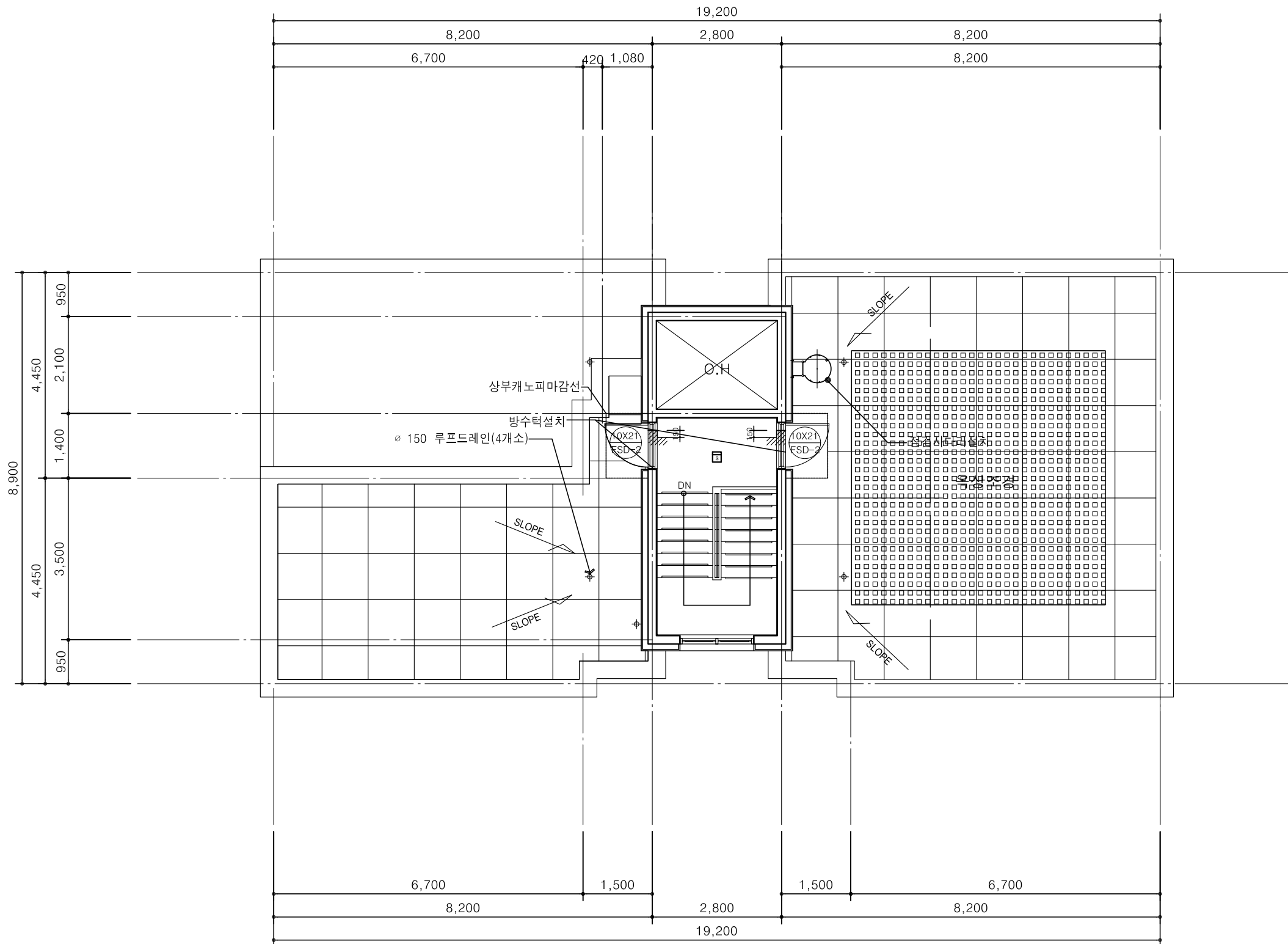
1 102동 옥탑층 동 평 면 도 축척: A3:1/100
