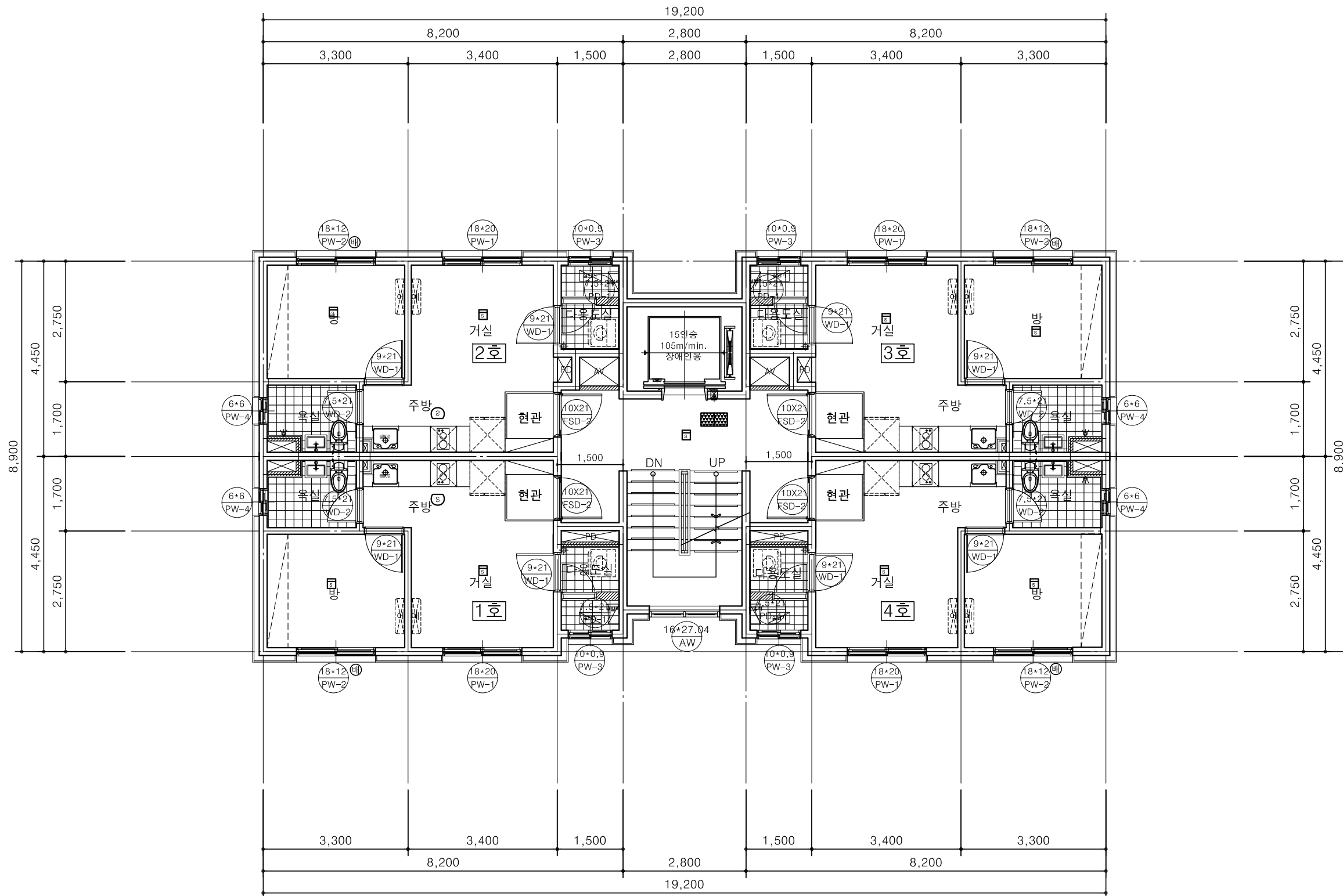
1 102동 2-8층 동 평 면 도 축척 : A3:1/100
