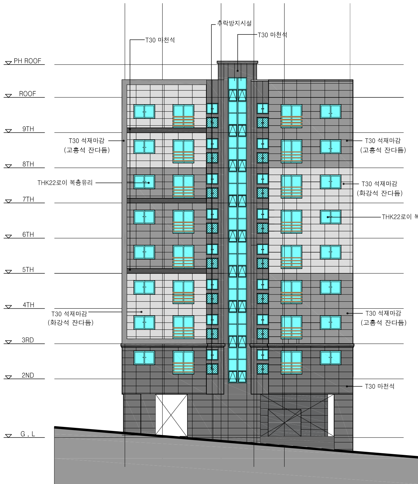
① 정 면 도 축척 : A3:1/200
