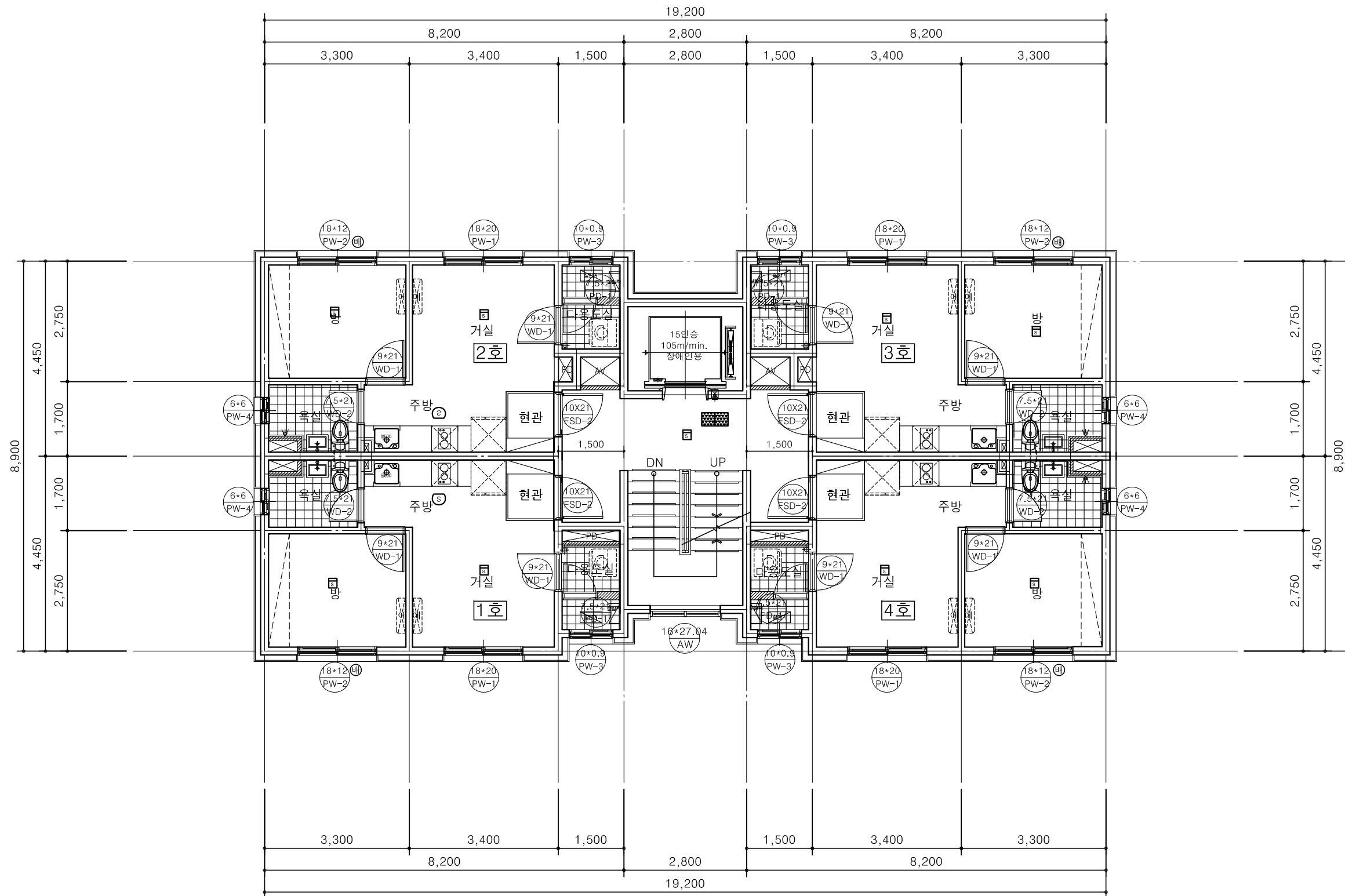
1 101동 2-9층 동 평 면 도 축척 : A3:1/100
