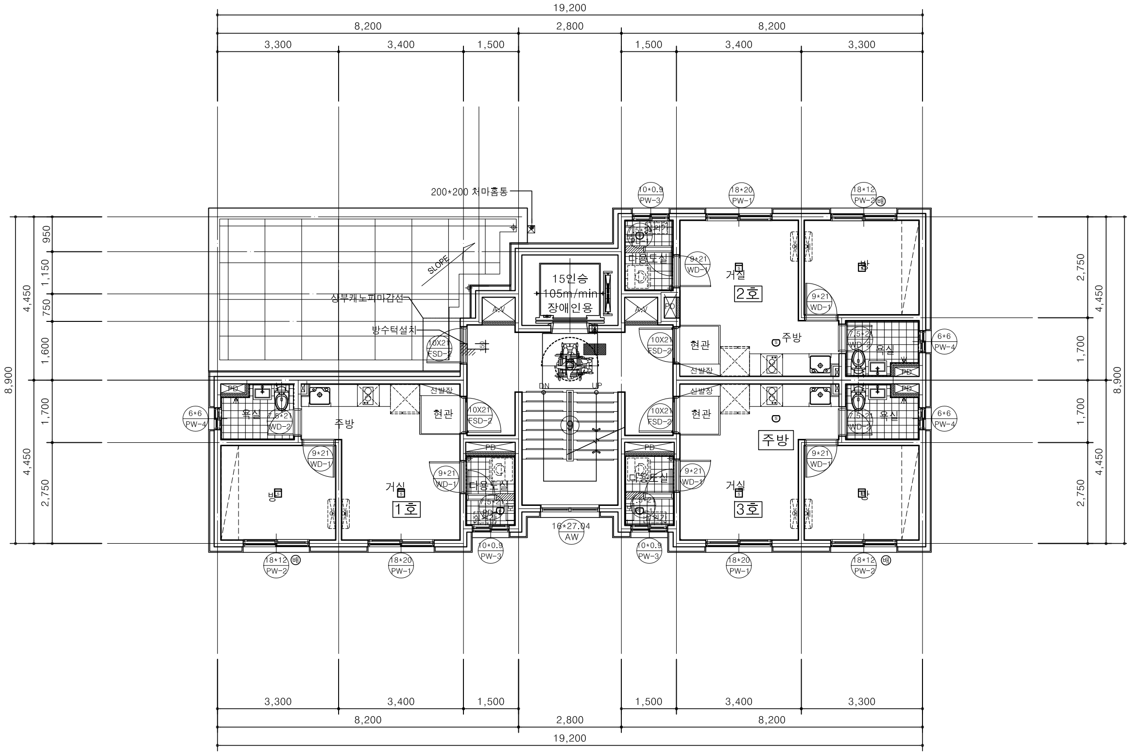
1 102동 9층 동 평 면 도 축척: A3:1/100
