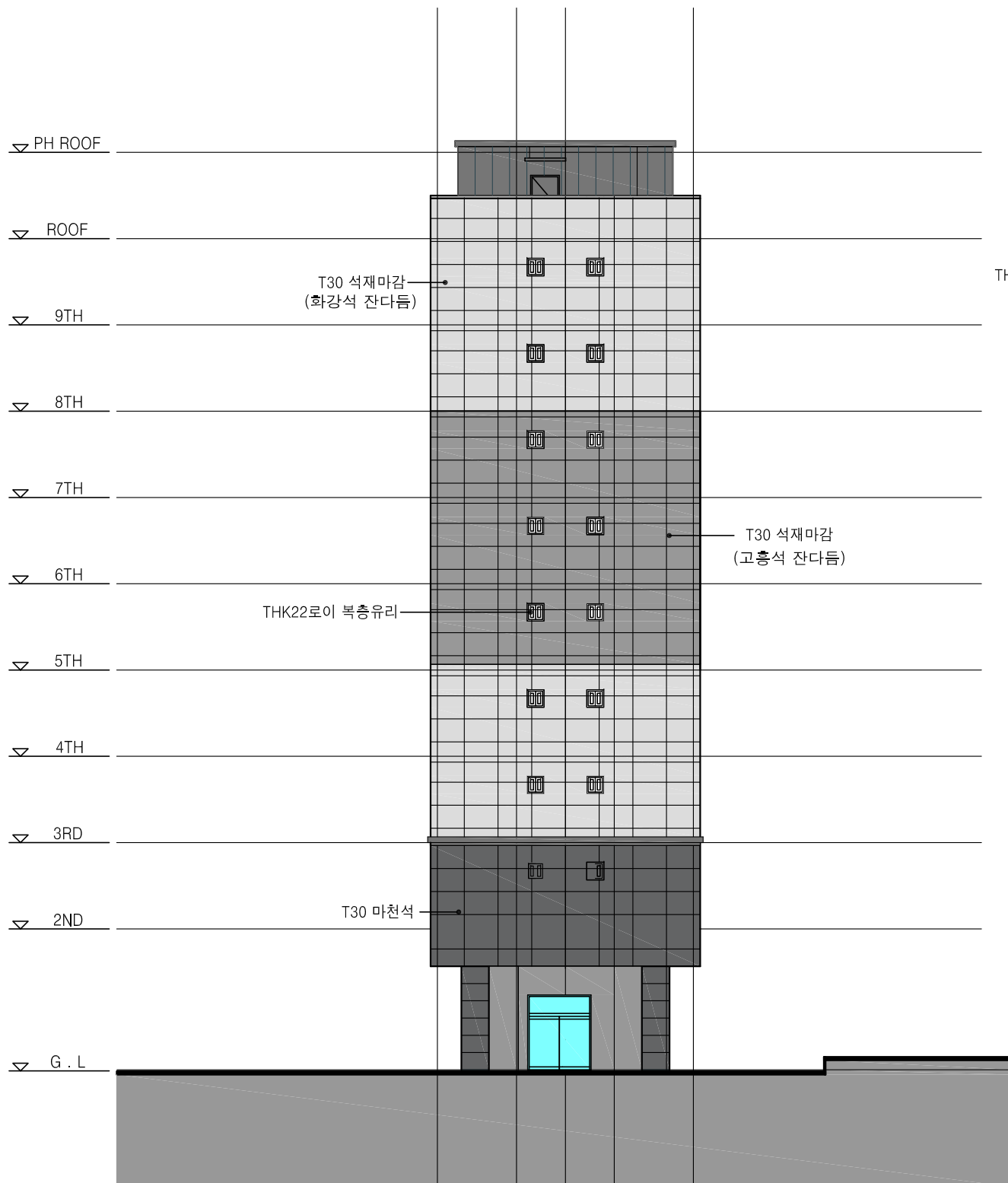
① 좌측면도 축척 : A3:1/200
