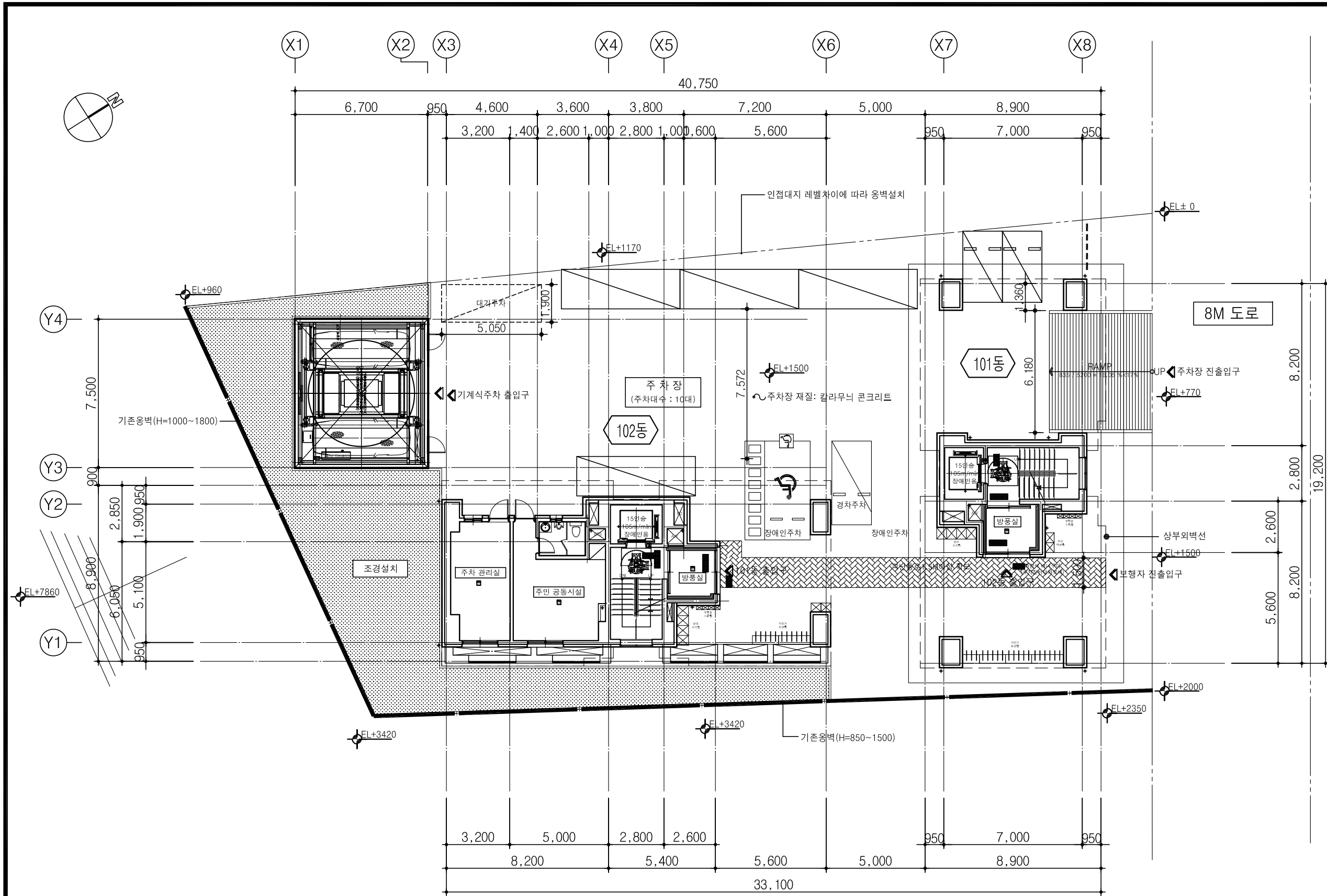
1 지상 1층 평면도 축척 : A3:1/200
